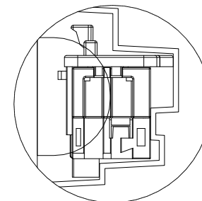
DETAIL: B 5:1
