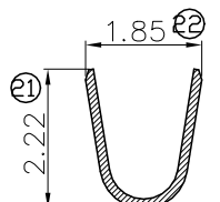
剖视图 B-B 比例 1:1
