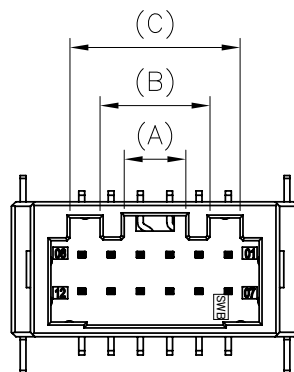
2*06 Pin
